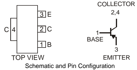
SOT89-3L
